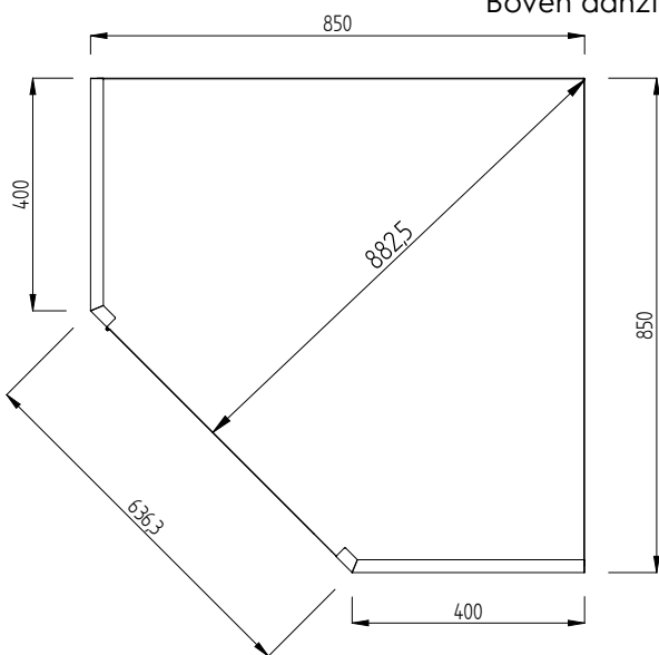
Boven aanzicht
